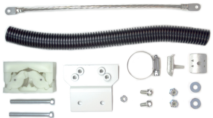
12A3 Cable Clamp for 0.25"-1.25" Diameter Cable P/N: 108-527-423
